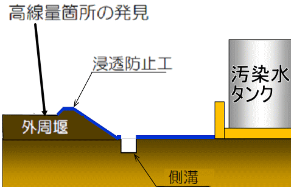
図一1 福島第一原発の汚染水タンクの堰の構造
