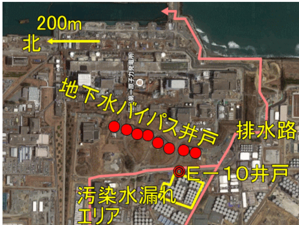
図一2 汚染水漏れを起こしたエリア
