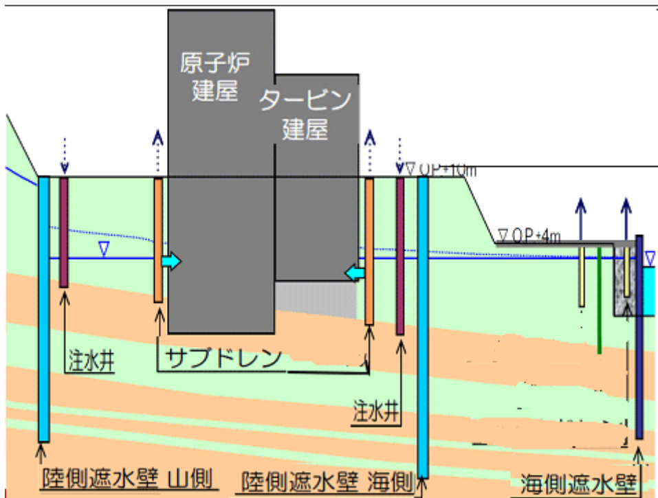
図一2 東電が実施を計画している汚染水抑制対策
