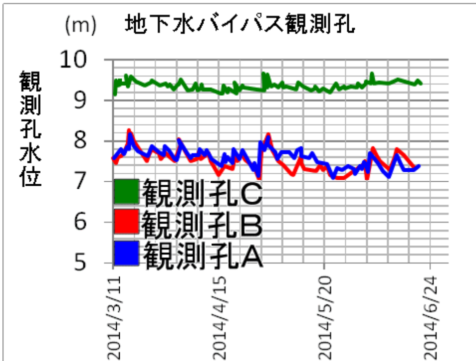
図-4 地下水バイパス用観測孔の水位
