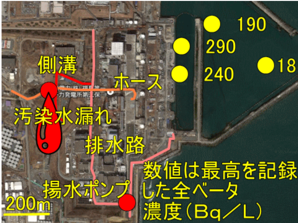
図一1 5月29日の汚染水漏れ箇所
