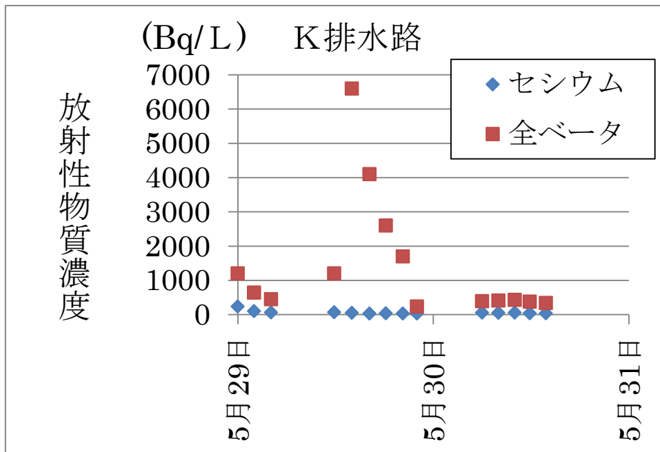
図一2 K排水路の放射性物質濃度
