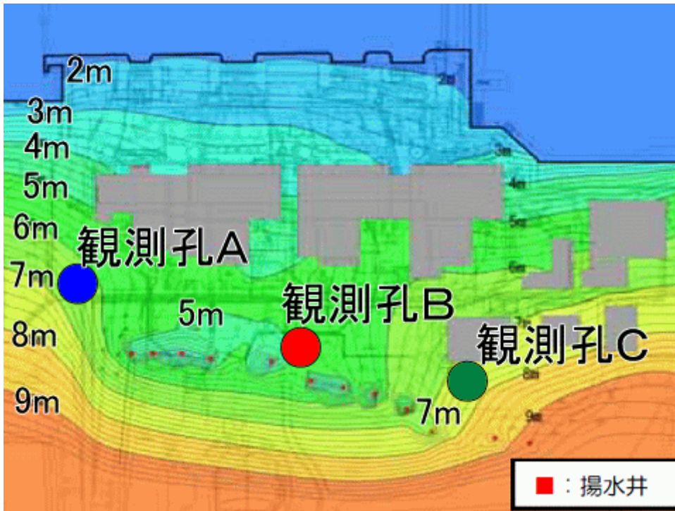
図-3 地下水バイパス稼働後の水位予測
