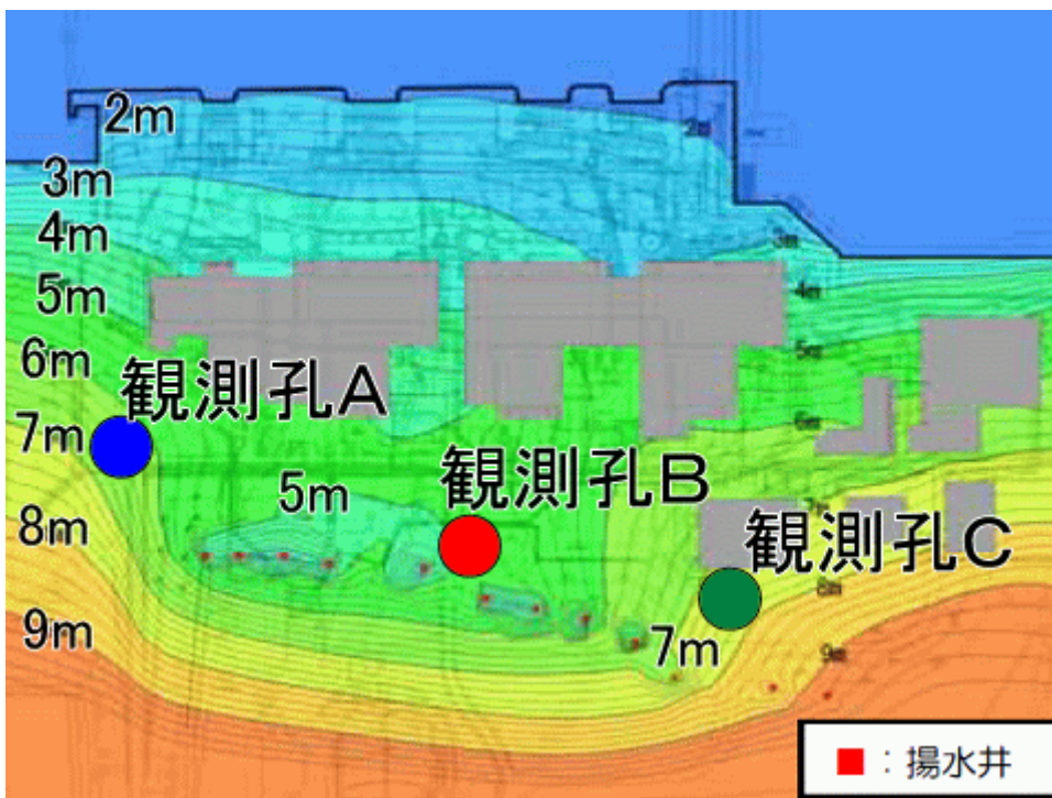
図一6 地下水バイパス稼働後の水位予測
