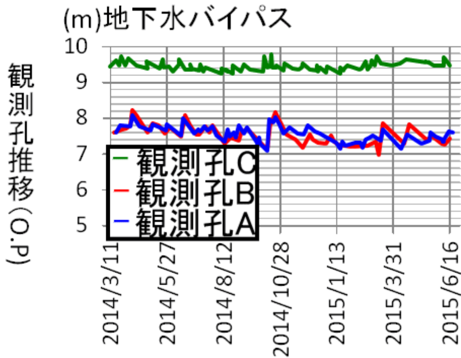
図一七 地下水バイパス用観測孔の水位
