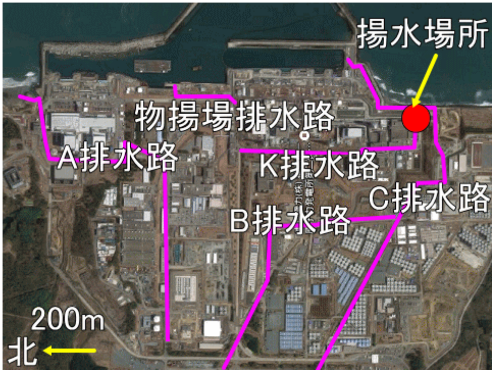
図一 3 福島第一原発内の排水路
