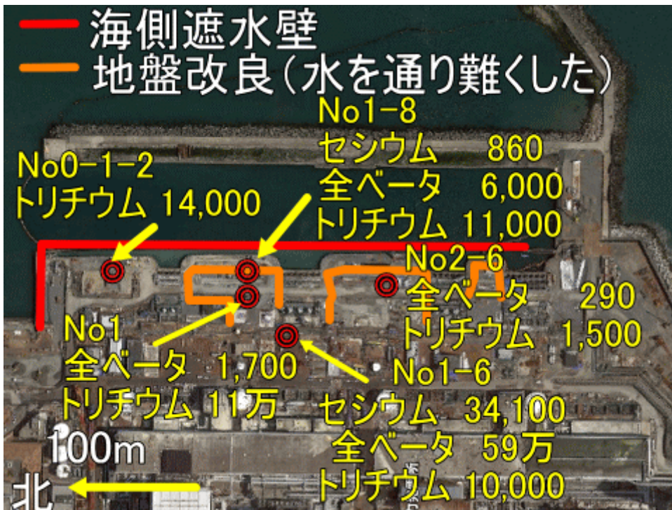
図一9 海岸付近の井戸の放射性物質濃度
