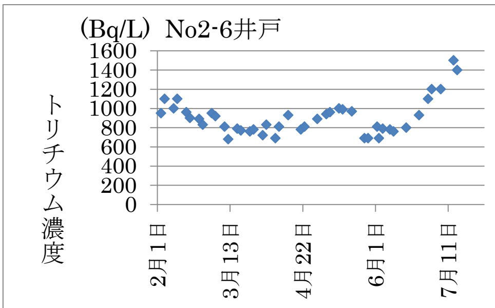
図一10 No2-6井戸のトリチウム濃度
