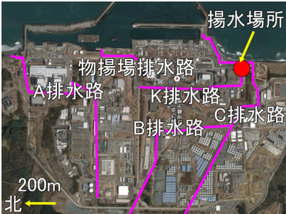
図一 1 1 福島第一原発内の排水路
