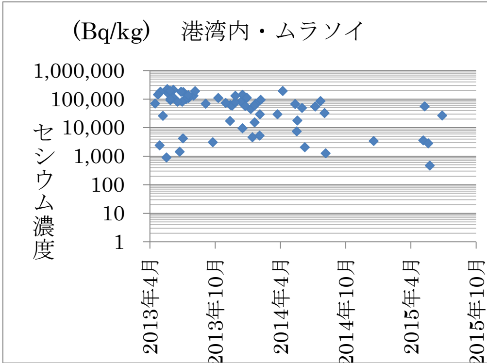
図一五 福島第一原発港湾内のムラソイのセシウム濃度
