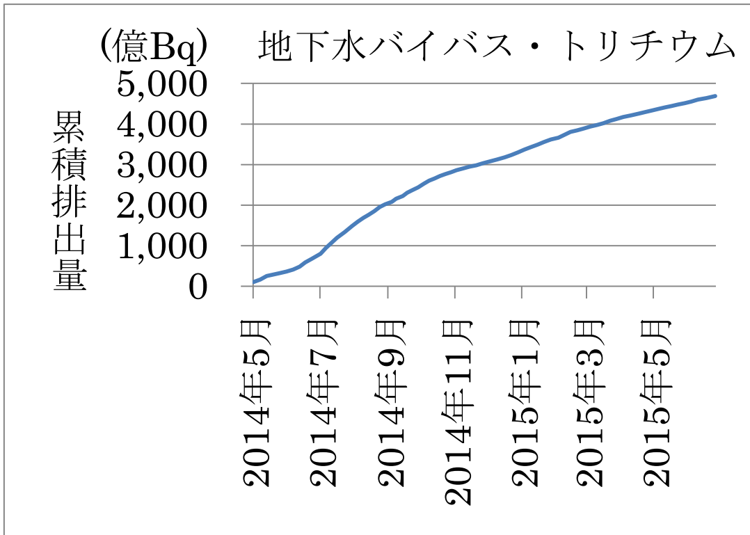
図一八 地下水バイパスの累積のトリチウム放出量
