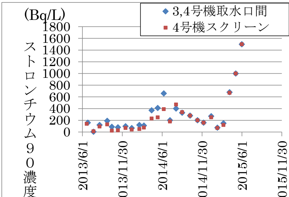
図一 4 3,4号機取水口間と4号機スクリーンのストロンチウム90濃度
