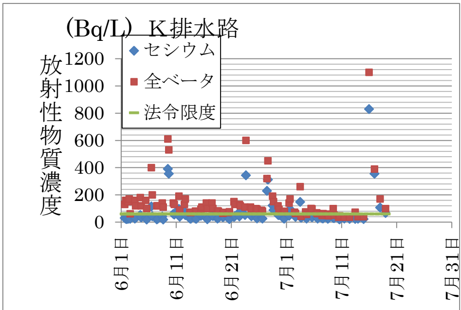
図一 1 2 K排水路の放射性物質濃度
