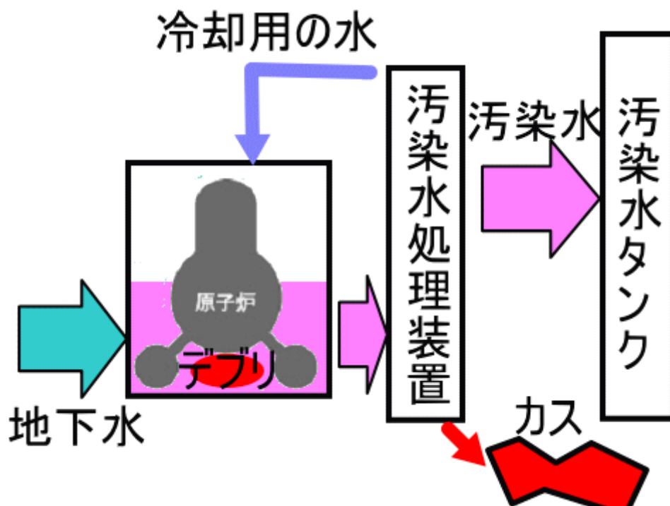
図一5 福島第一の汚染水処理の流れ
