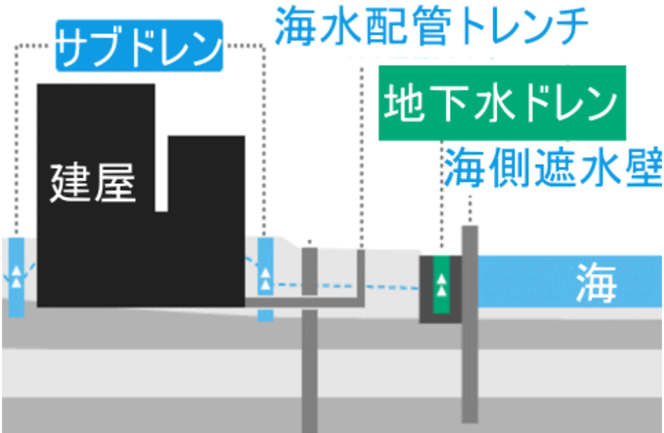
図一 1 0 サブドレンの概要
