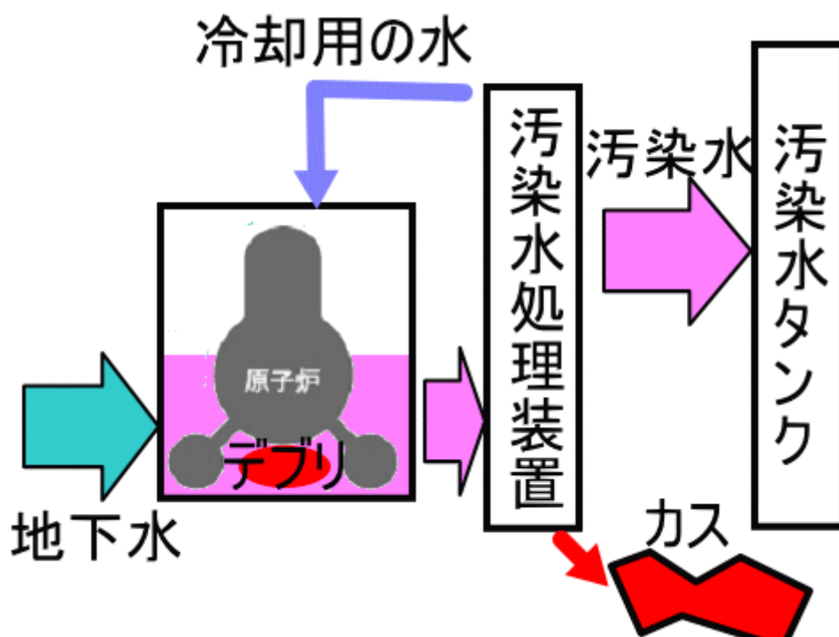
図一1 福島第一の汚染水処理の流れ
