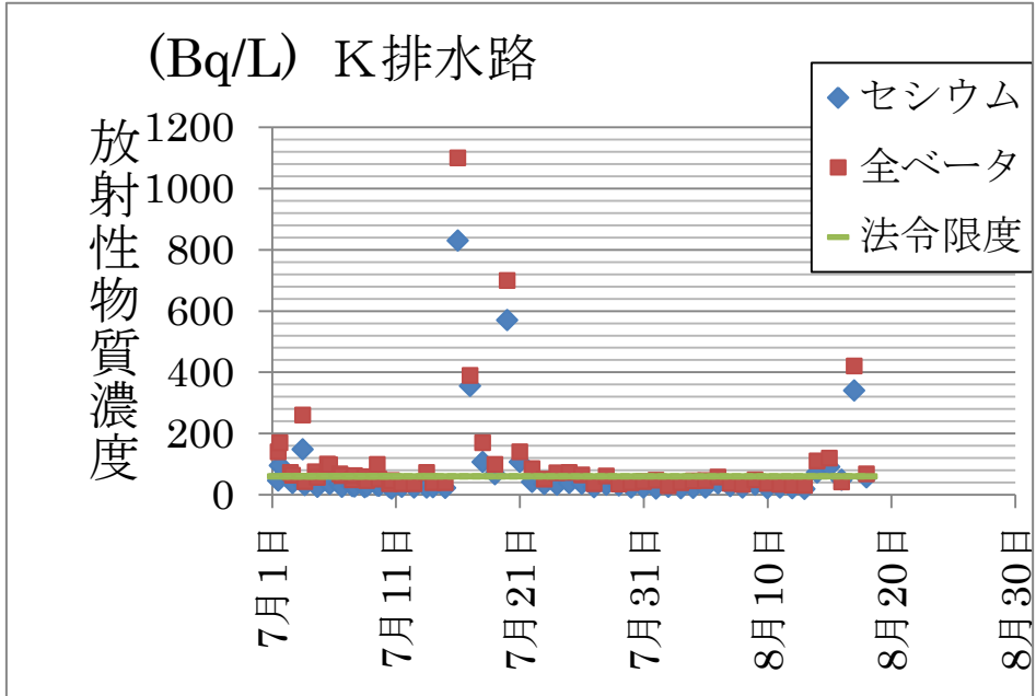
図-5 K排水路の汚染水濃度
