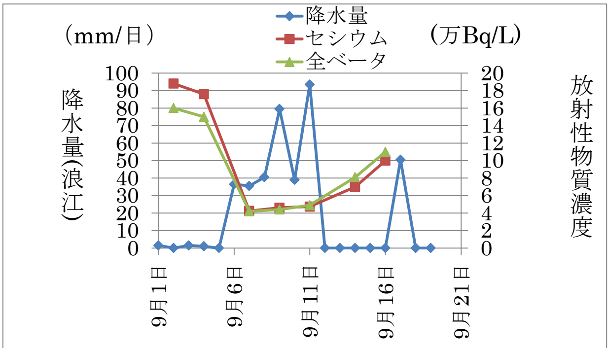
図一6 1号機放水路の放射性物質濃度と降水量
