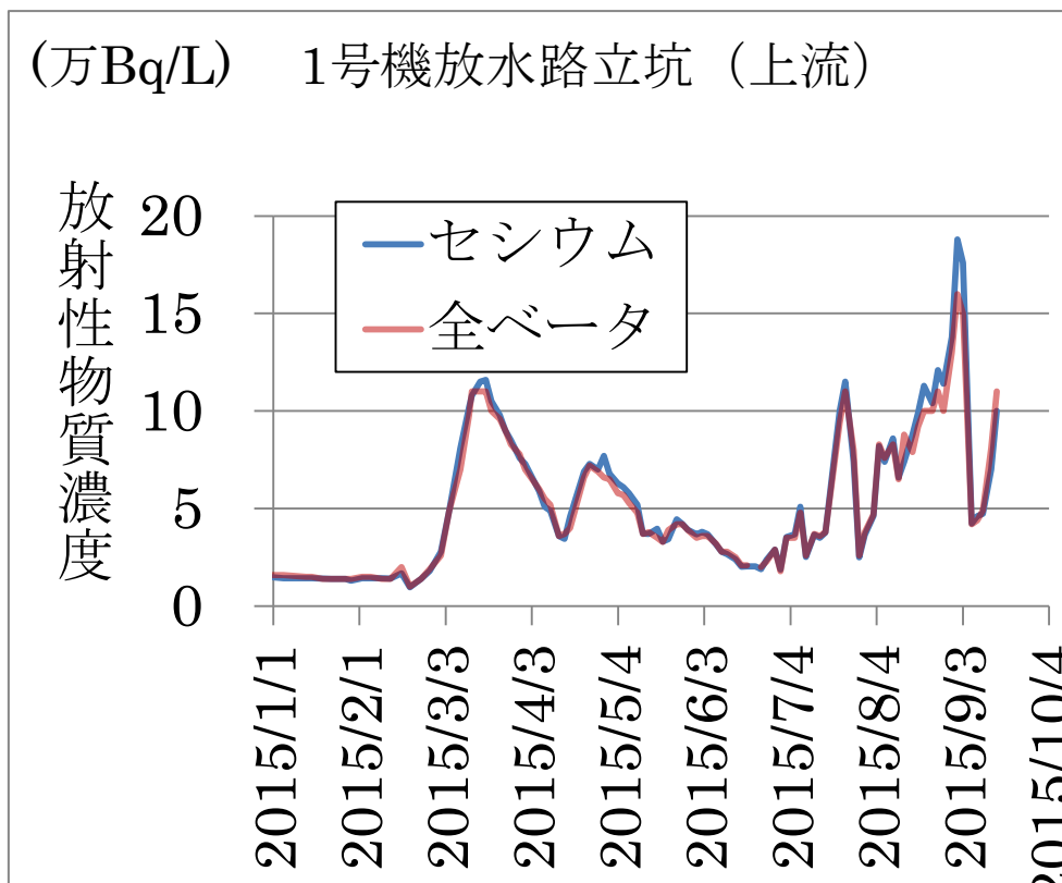
図一2 1号機放水路の放射性物質濃度 (その1)
