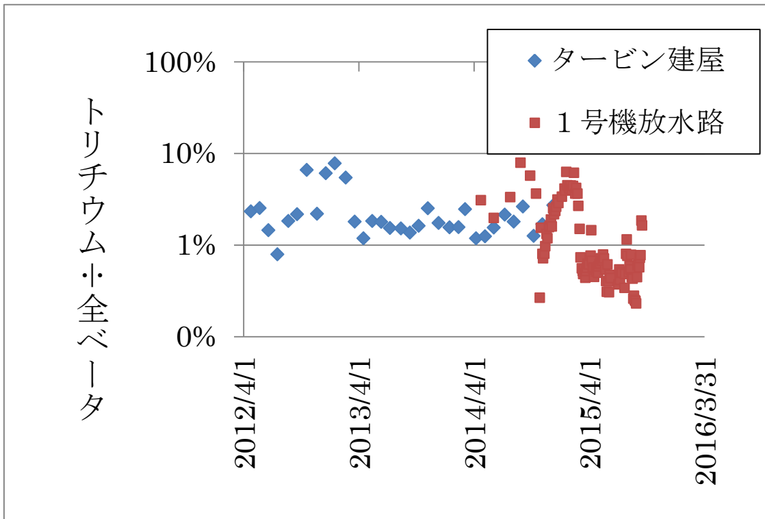
図一5 全ベータに対するトリチウムの割合
