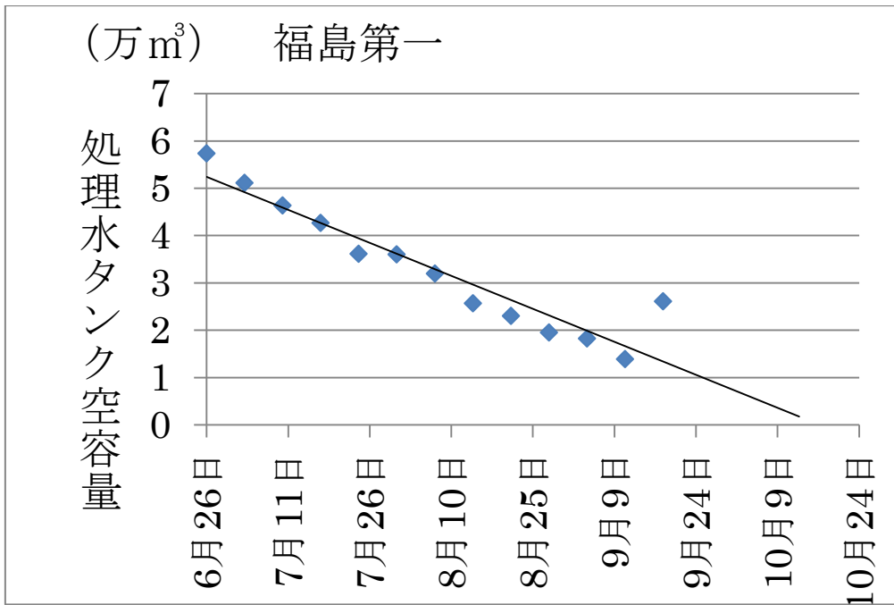
図一6 処理水タンクの空き容量
