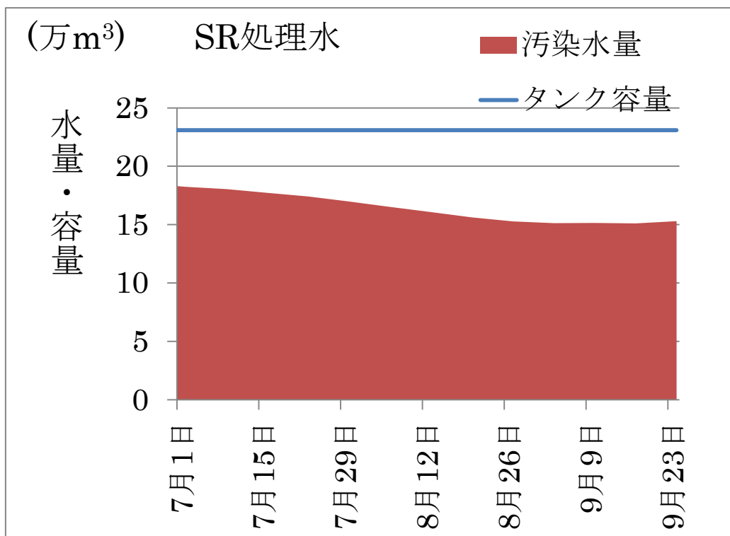
図一 4 SR 処理水の (汚染) 水量とタンク容量
