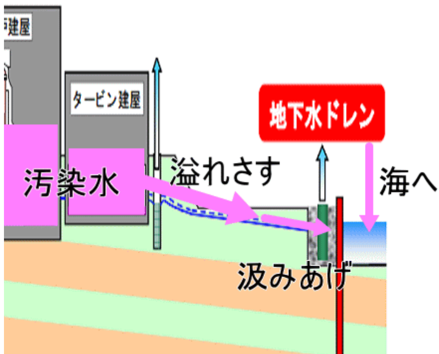
図一 9 新しい汚染水抑制手段
