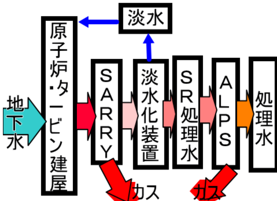
図一 3 福島第一原発の汚染水処理の流れ
