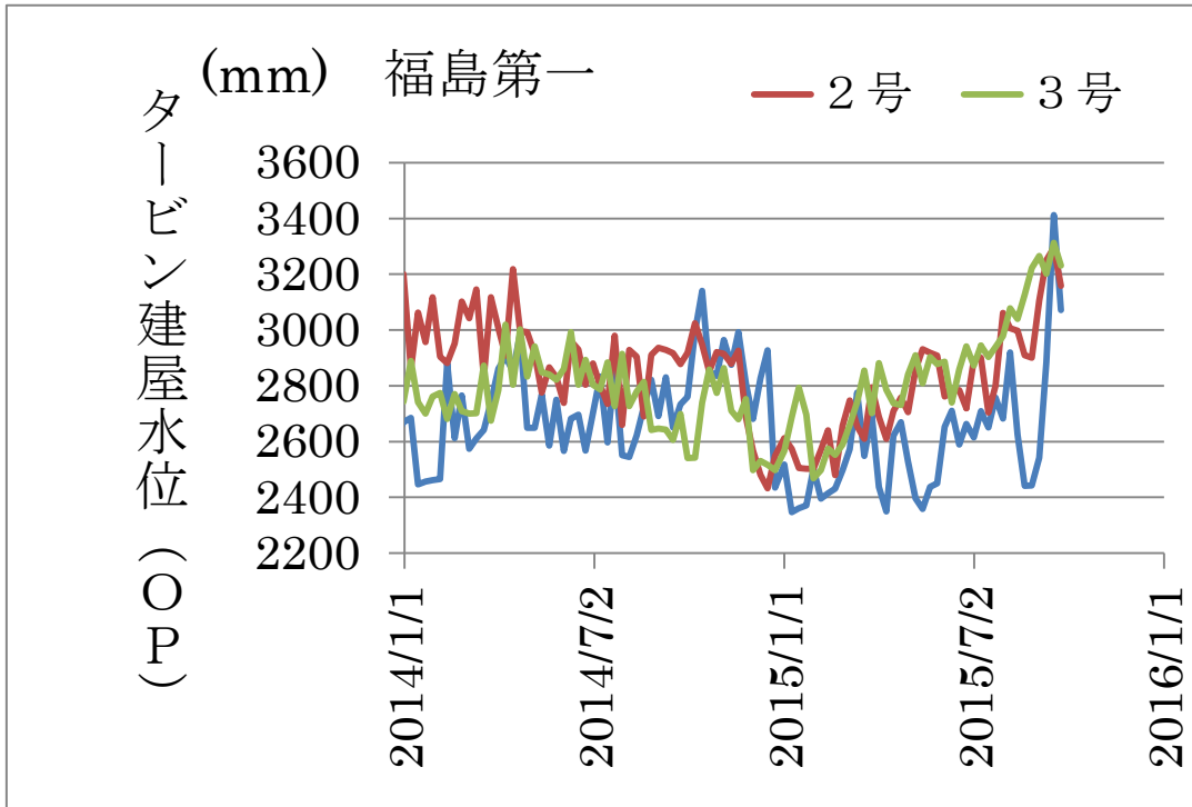
図一七 タービン建屋内の汚染水水位
