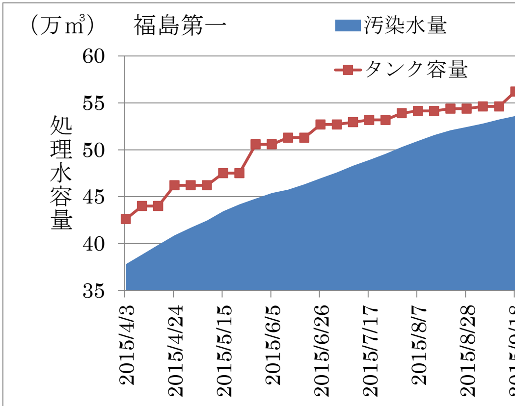
図一5 処理水量とタンク容量
