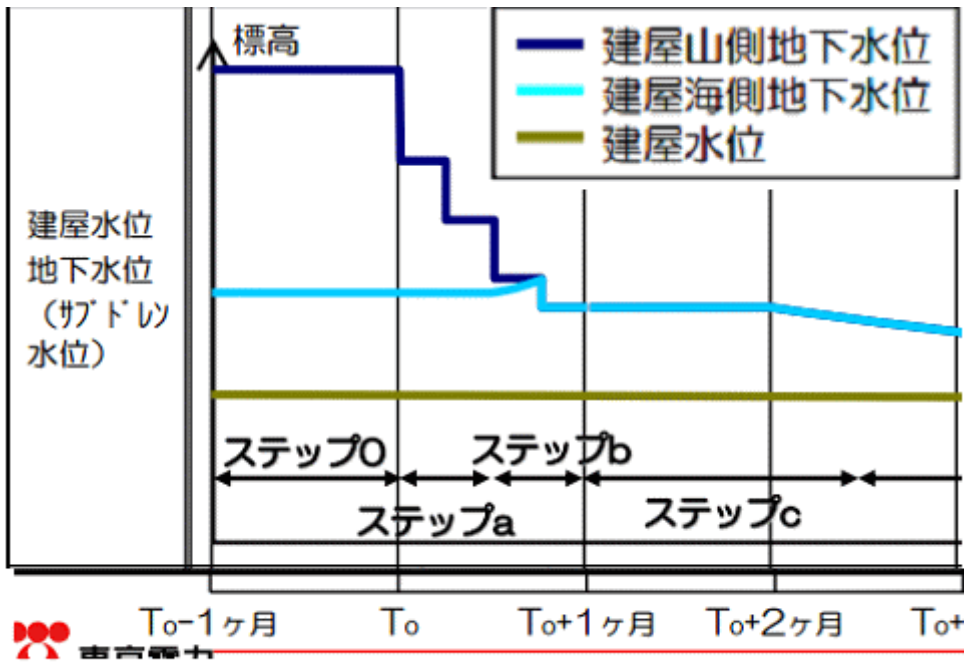
図-1 サブドレン稼働後の水位予測
