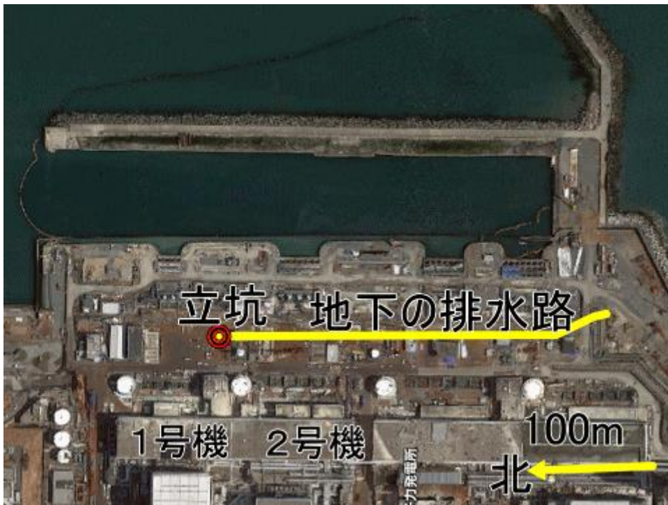
図一 1 2 タービン建屋と海の間排水路
