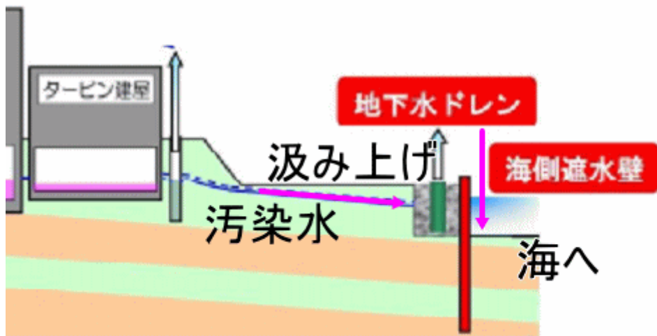
図-5 海側遮水壁と地下水ドレン
