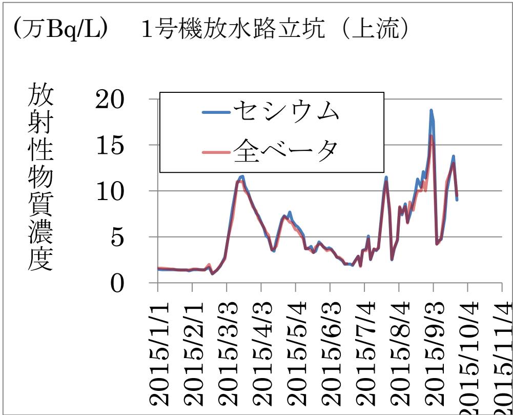
図-13 タービン建屋と海との放水路の放射性物質濃度
