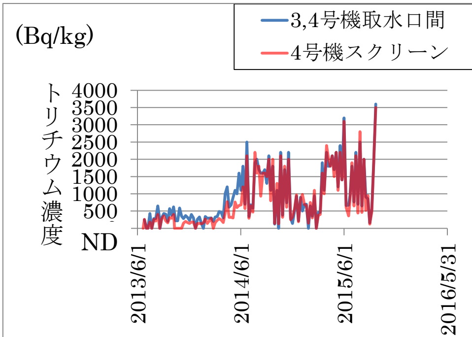
図一4 3,4号機取水口間と4号機スクリーンのトリチウム濃度
