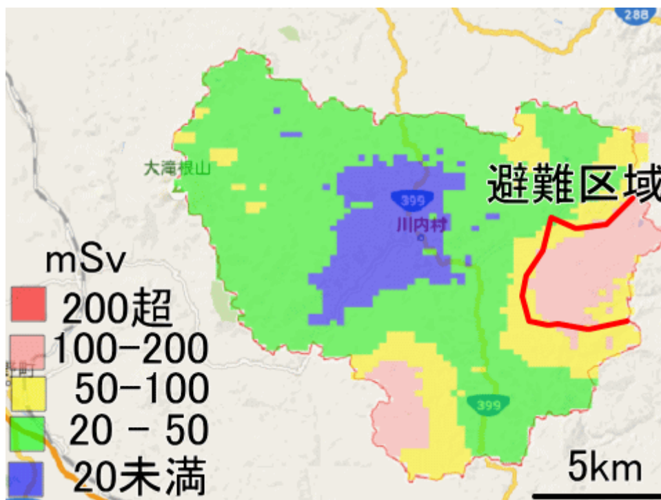
図一1 帰還後30年での被ばく線量
