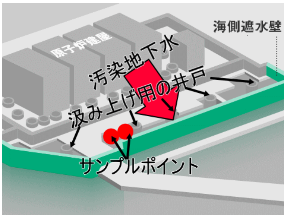
図一1 海側遮水壁の概要
