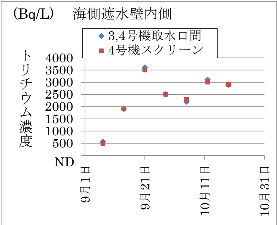
図一3 海側遮水壁内側（3,4号機取水口間および4号機スクリーン）のトリチウム濃度
