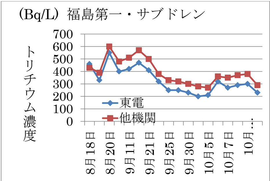
図一4 サブドレン放流水のトリチウム濃度
