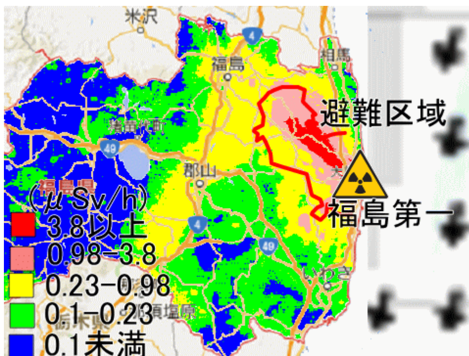
図-2 半減期から計算される放射線量
