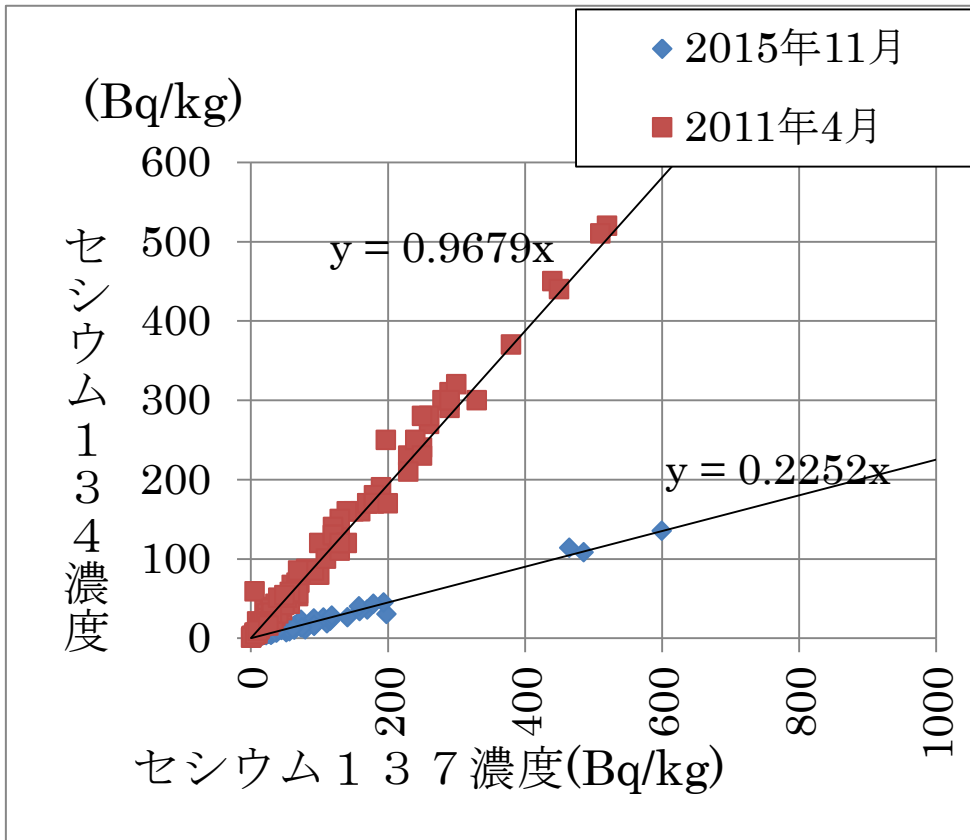
図-3 セシウム137に対するセシウム134の割合
