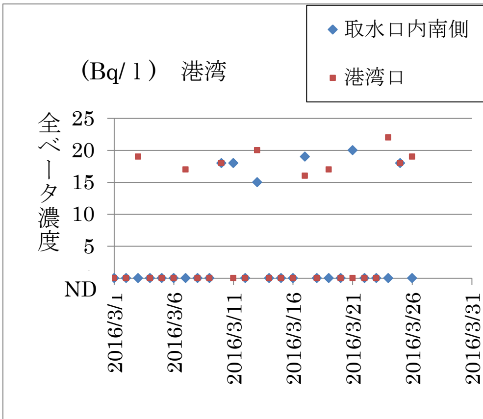
図一 4 港湾口と1~4号機取水口内南側の全ベータ濃度
