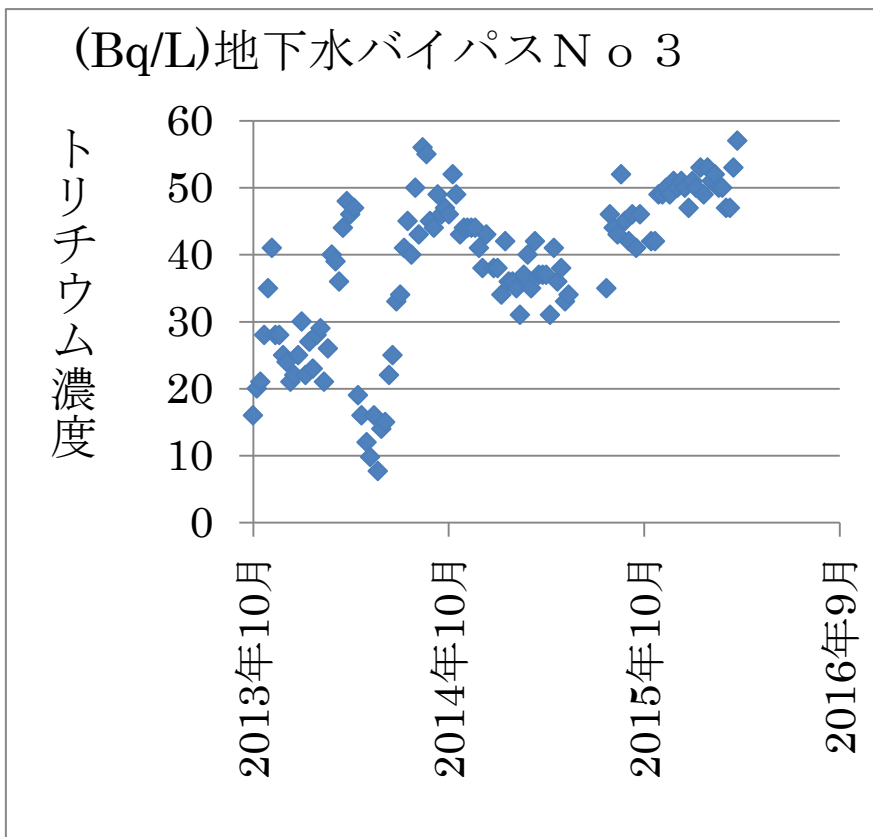
図一6 地下水バイパス井戸No.3のトリチウム濃度
