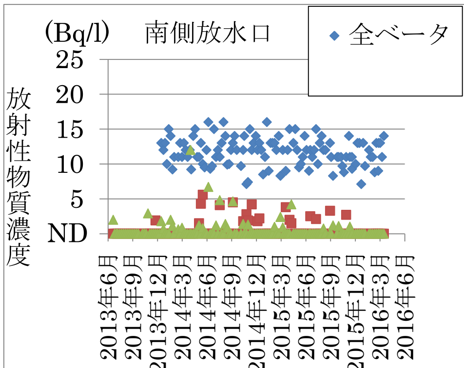
図一2 南放水口北側の放射性物質濃度
