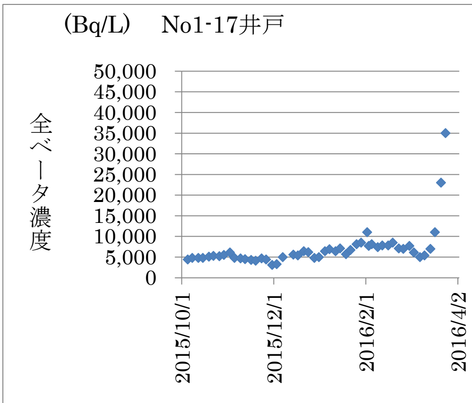
図一八 No17井戸の全ベータ濃度
