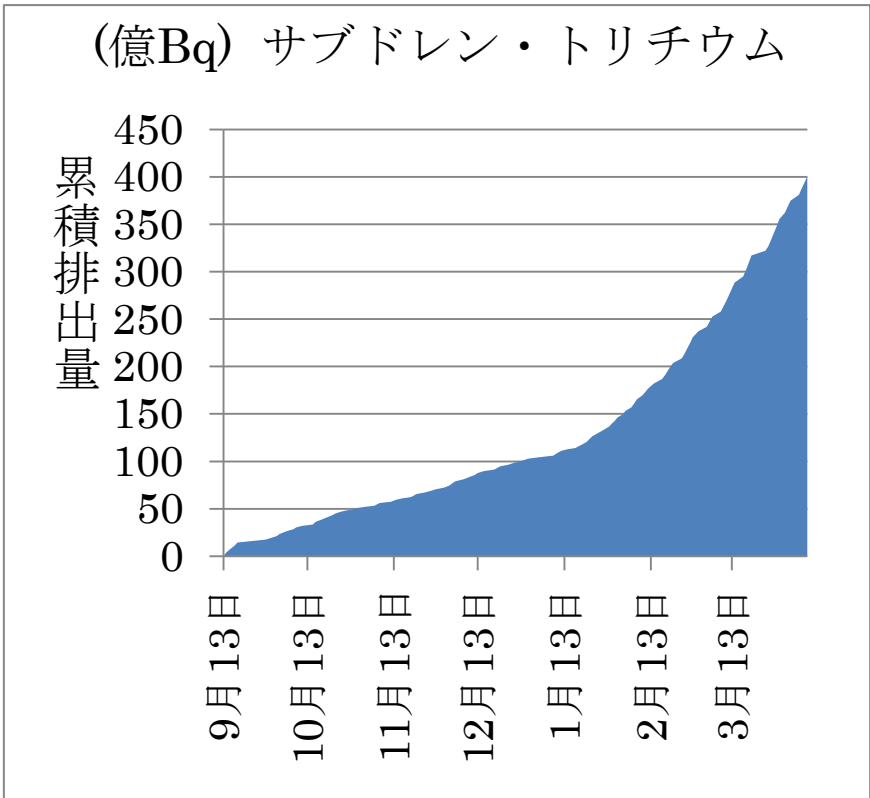
図一6 サブドレンのトリチウム累積排出量
