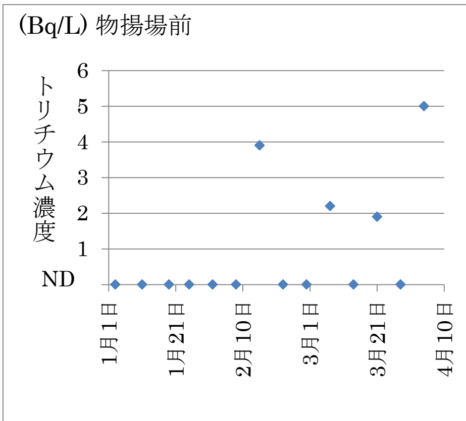
図一八 物揚場前のトリチウム濃度
