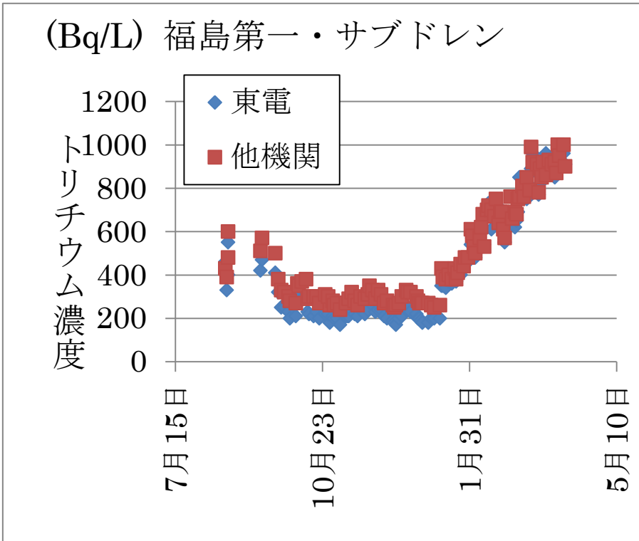
図一5 サブドレン排水のトリチウム濃度
