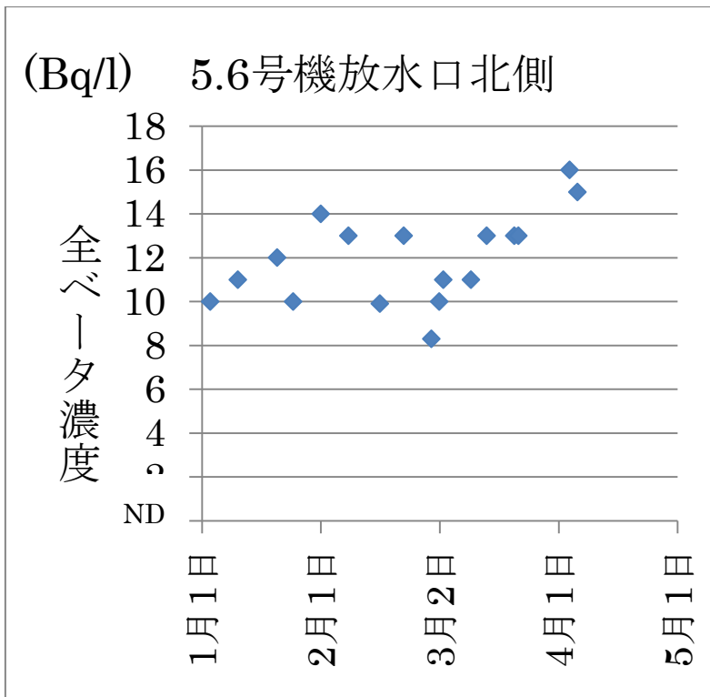
図一 2 5, 6号機放水口北側の全ベータ濃度
