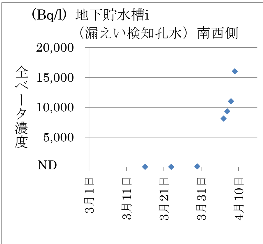
図-4 地下貯水槽 i (漏えい検知孔水) 南西側の全ベータ濃度
