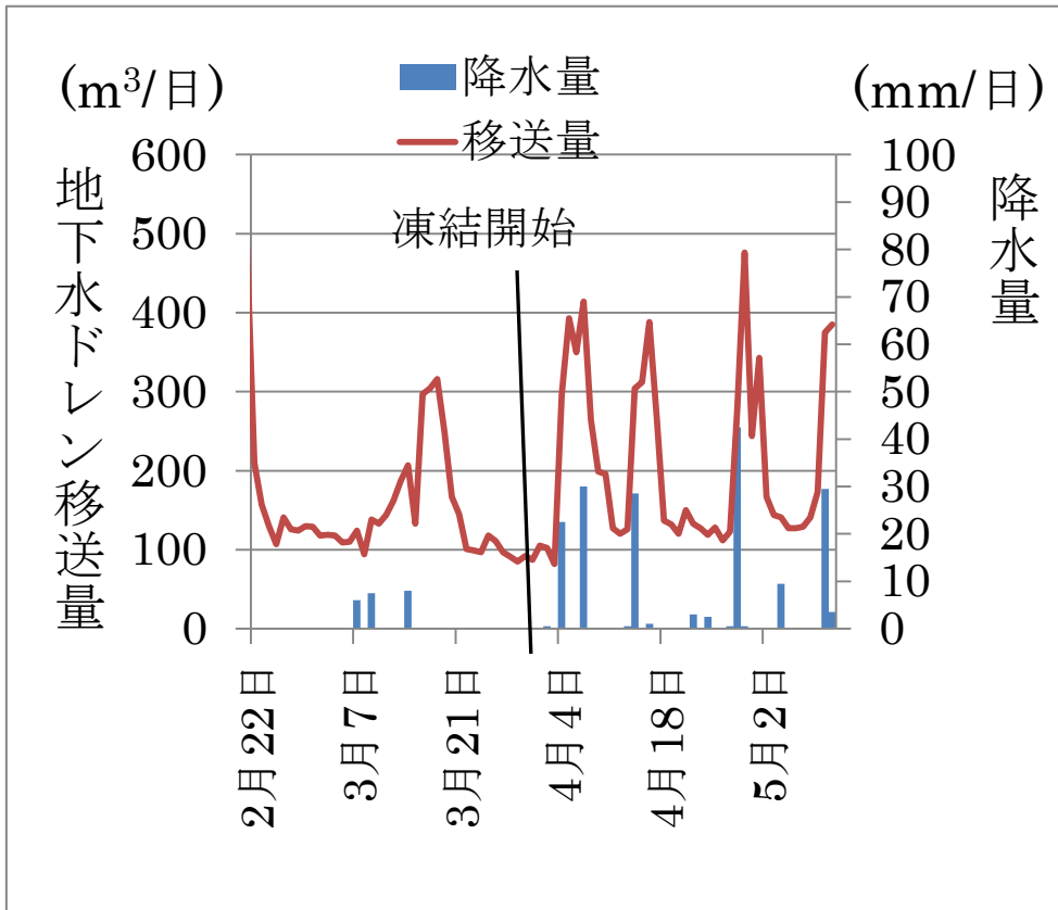
図-9 地下水ドレン等からタービン建屋への移送量
